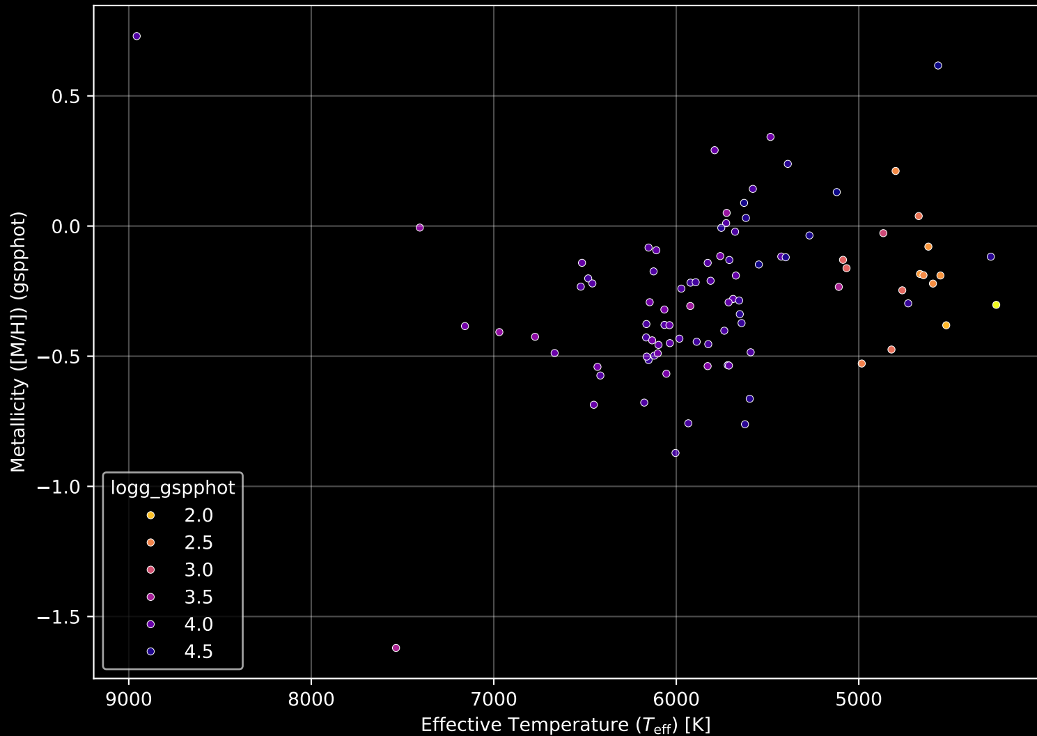
GALAH DR4 Field: [7154] Stellar Population Parameters (n= 92)
