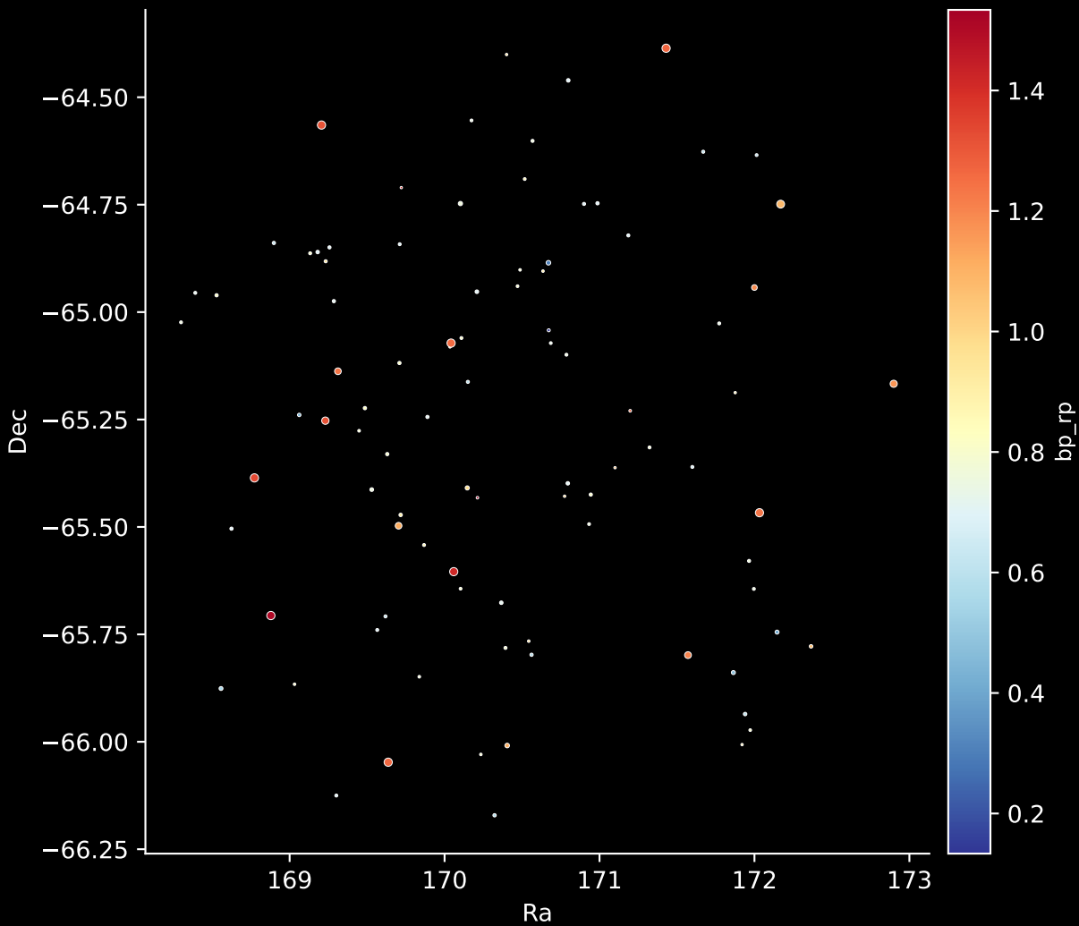
GALAH DR4 Field: [7154] Stars: 92
